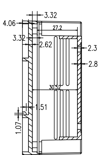
剖面 A-A
